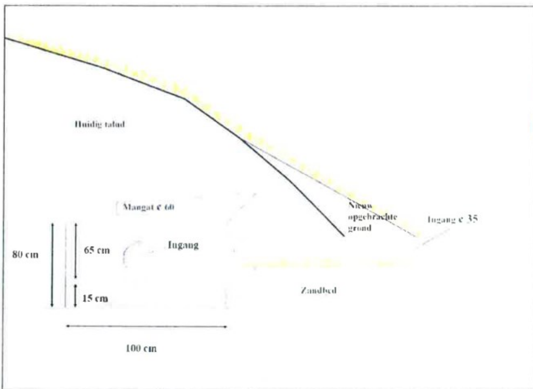
Figuur 12. Dwarsdoorsnede kunstburcht das.
